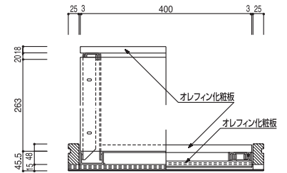
姿見付タイプ/スツールタイプ 平面図
